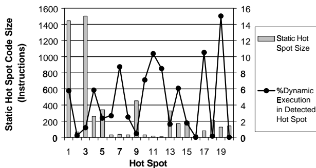
(b) PhotoDeluxe(A).
