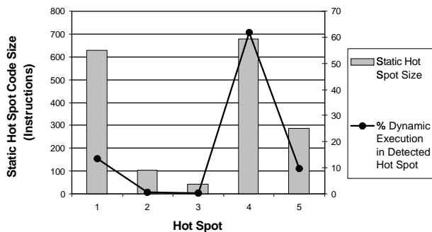
(a) 134.perl.
